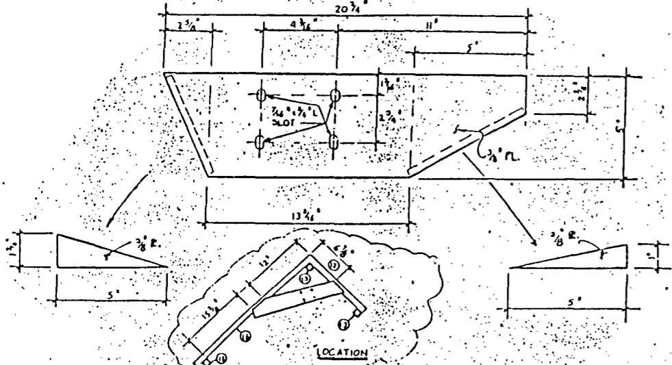
MOTOR MOUNTING BRACKET N.T.S.
