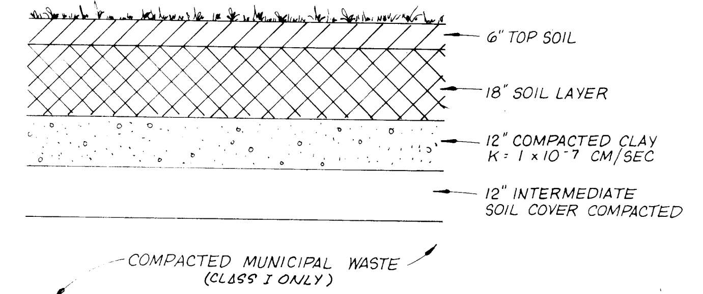
FINAL COVER - CLASS I & III N.T.S.
