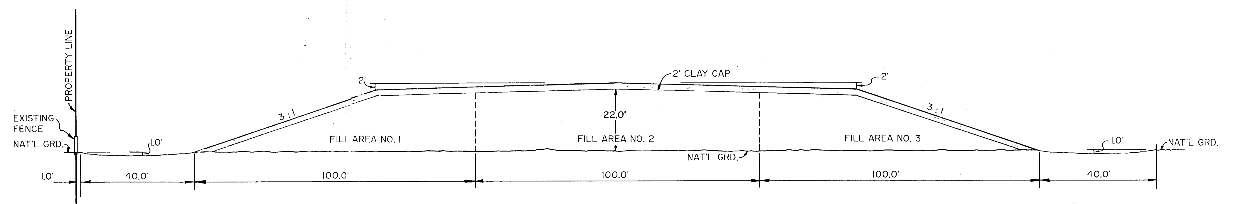
SECTION A-A
